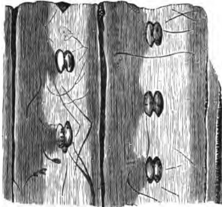
SIGILLARIA RENIFORMIS. (Nat. size.)
